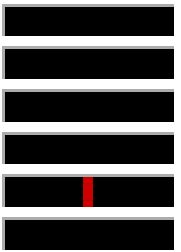
離下乾上
