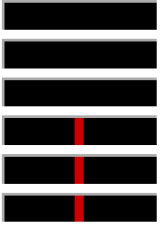
坤下乾上
