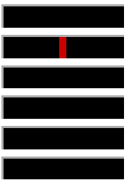
乾下離上
